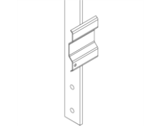
Attente applique GC60 ▼
